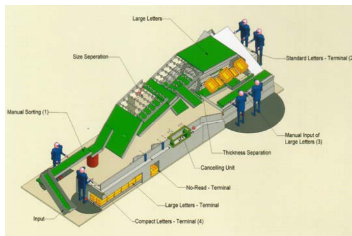
Prinzip der automatischen Brief-Frankierung mit manueller Vorsortierung
